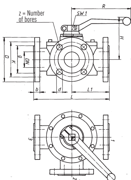
DN 50-100 ▲
